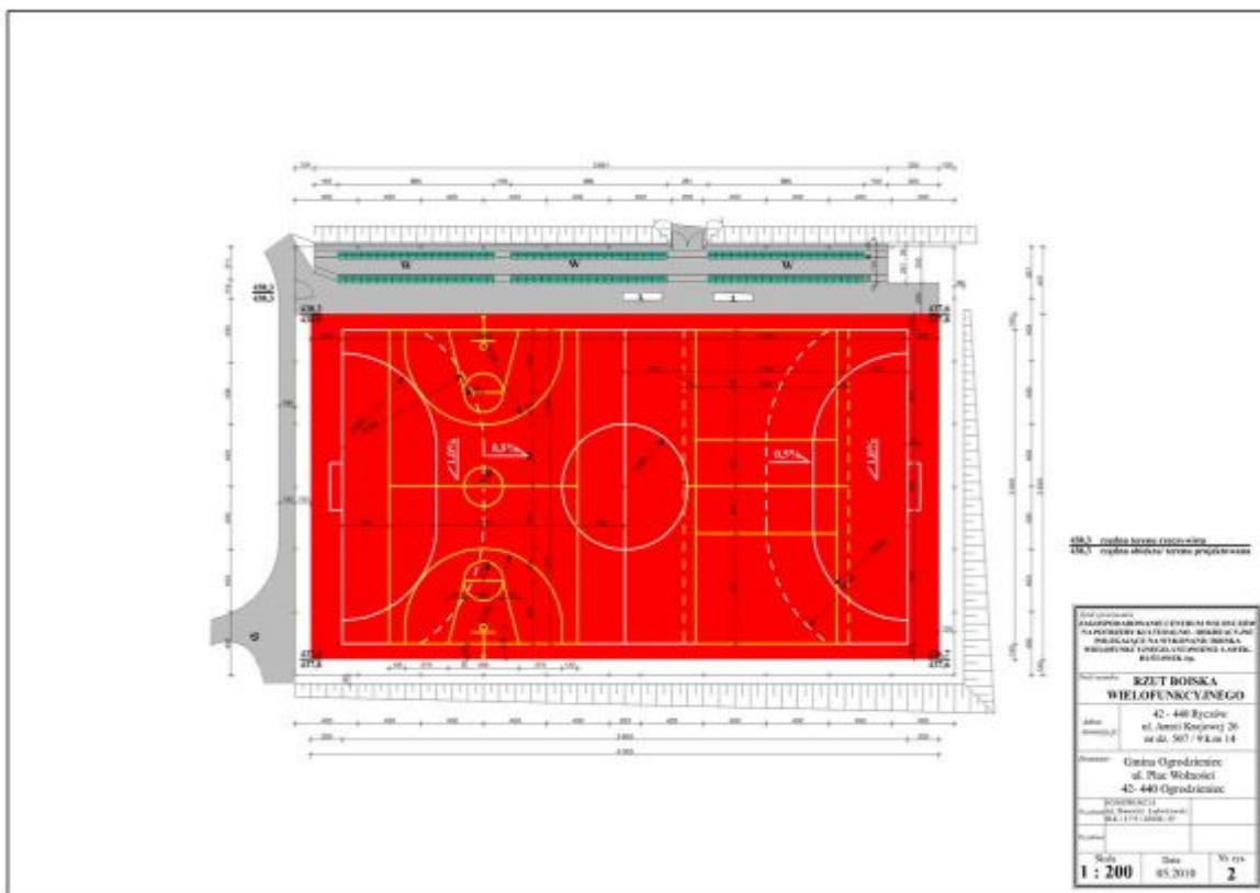
Fot.12. Projekt "Zagospodarowanie Centrum Wsi Ryczów na potrzeby kulturalno-rekreacyjnej" – rzut boiska wielofunkcyjnego
