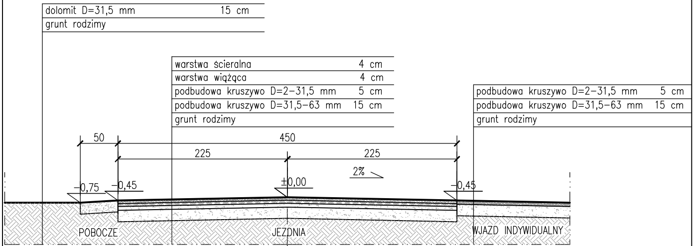
PRZEKRÓJ POPRZECZNY JEZDNI
