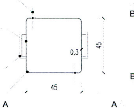
RZUT ŚCIAN URNY założona grubość ścian 3 mm
